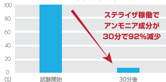
JEM1467脱臭性能試験の結果
